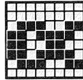
176 &HBO &X10110000
